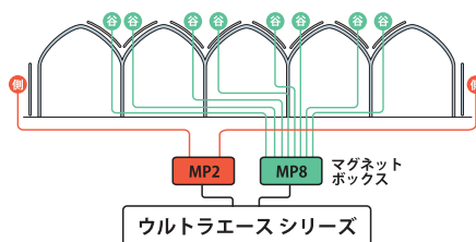
例② 側面換気+谷面換気 駆動モーター × 10台
